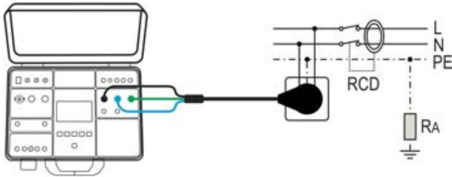
Fig. 42: Connexion du câble d'essai Schuko
