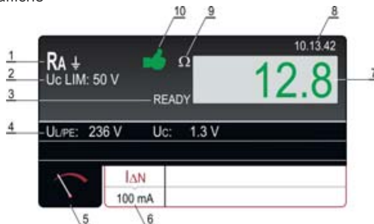
Fig. 54: Page-écran des résultats des essais RA
