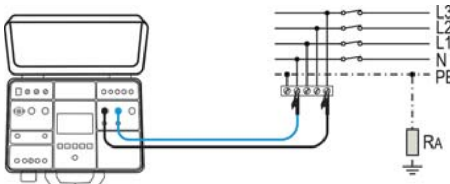
Fig. 47: Connexion des bornes d'essai au câblage testé pour mesure BOUCLE L/N
