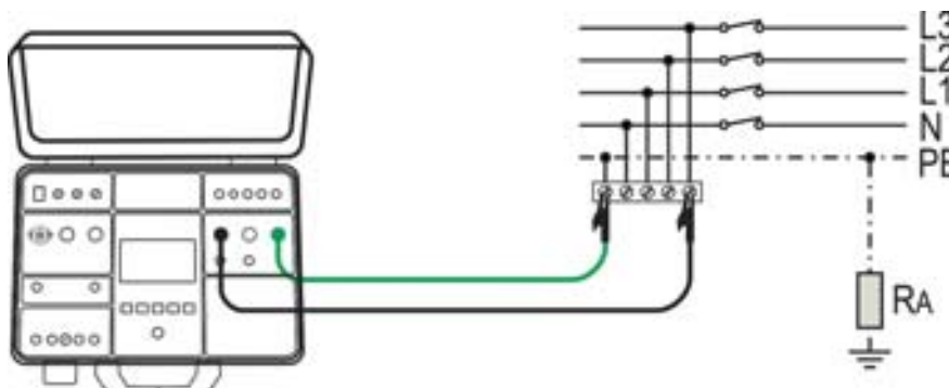
Fig. 48: Connexion des bornes d'essai au câblage testé pour mesure BOUCLE L/PE
