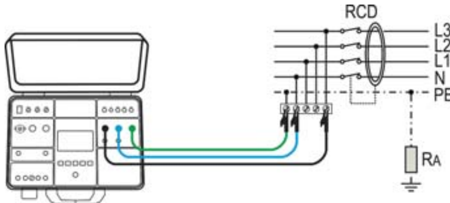
Fig. 53: Connexion des bornes de mesure au câblage testé
