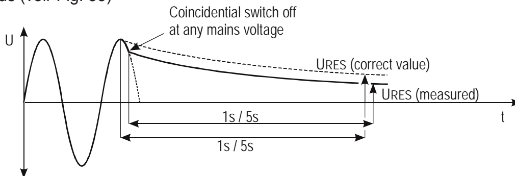
Fig. 55: Schéma de décharge en mode Lineaire
