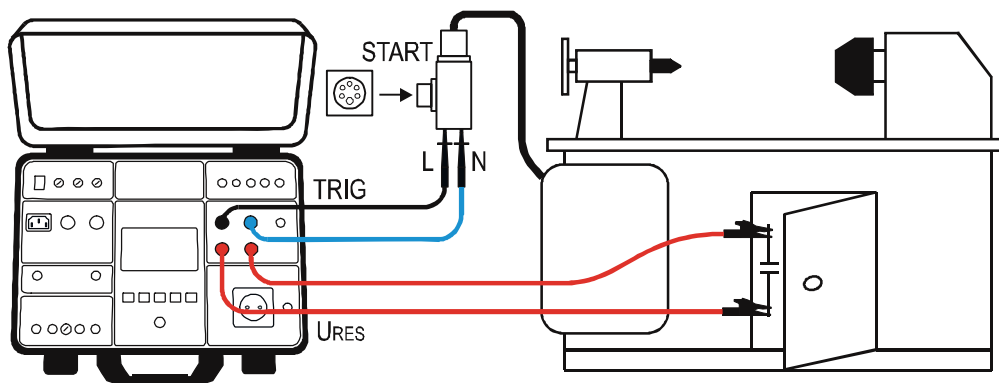
Fig. 58: Connexion pour mesure URES INT sur les machines connectées 1P/3P
