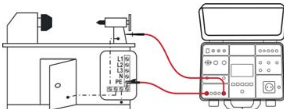
Fig. 27: Connexion des bornes de mesure dans la fonction RPE-2WIRE
