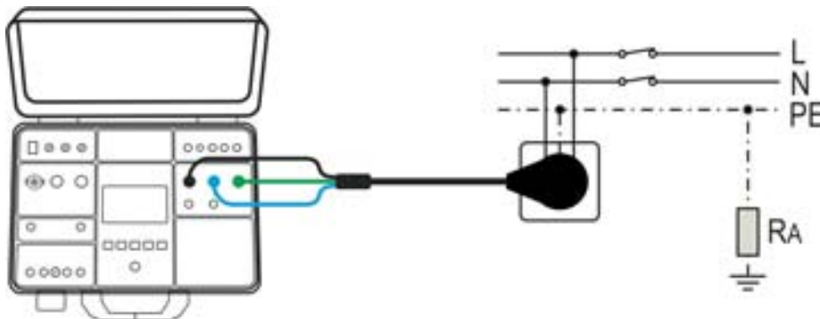
Fig. 46: Connexion à la prise schuko pour mesure BOUCLE L/N ou BOUCLE L/PE
