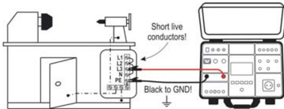
Fig. 33: Connexion des bornes de mesure MΩ
