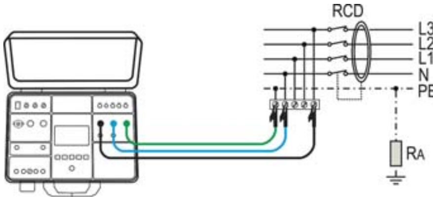
Fig. 43: Connexion des bornes de mesure
