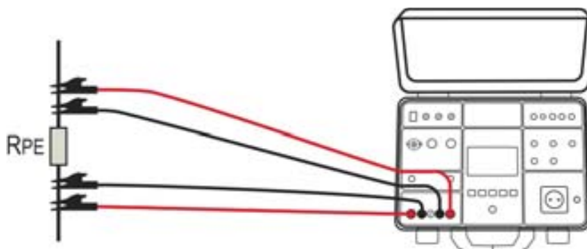
Fig. 30: Connexion des bornes de mesure dans la fonction RPE-4WIRE
