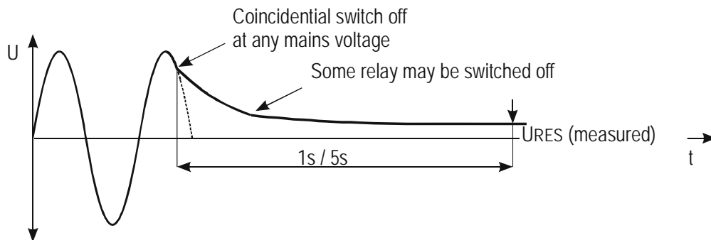
Fig. 56: Schéma de décharge en conditions Non Lineaire
