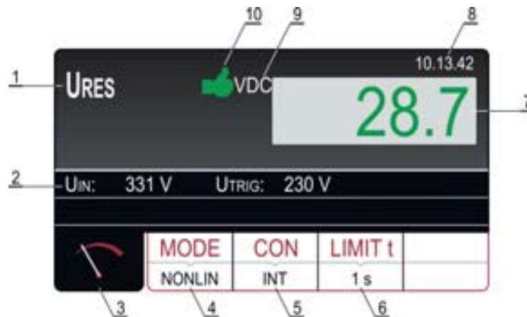
Fig. 61: Page-écran des résultats des essais URES
