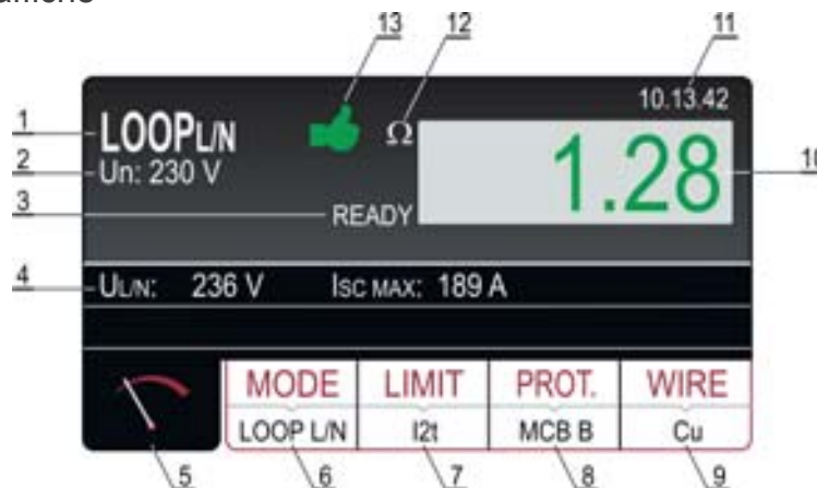
Fig. 50: Page-écran avec le résultat du test LOOP
