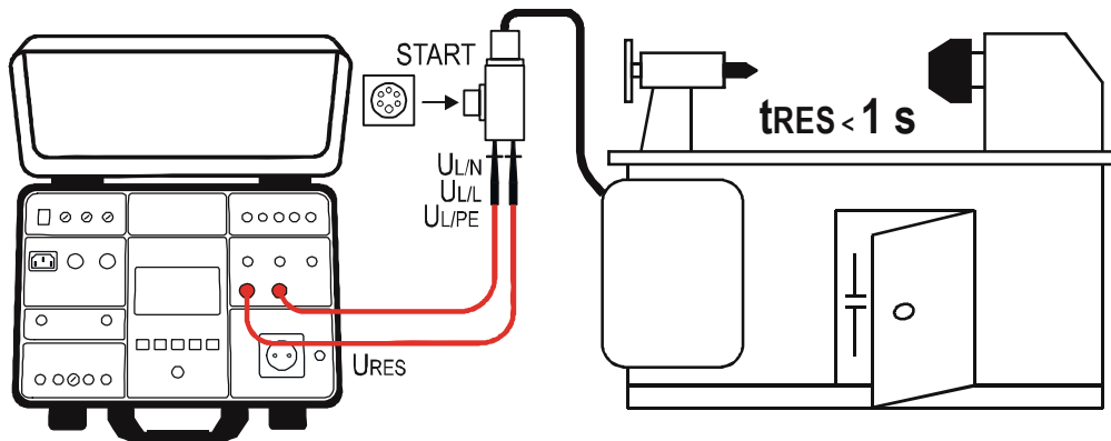
Fig. 60: Connexion des bornes de mesure dans la mesure URES PLUG
